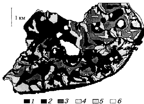
Рис. 1. Карта сезонного чистого потока CO_2 в ландшафте типичной субарктической тундры Северо-Западного Таймыра.
